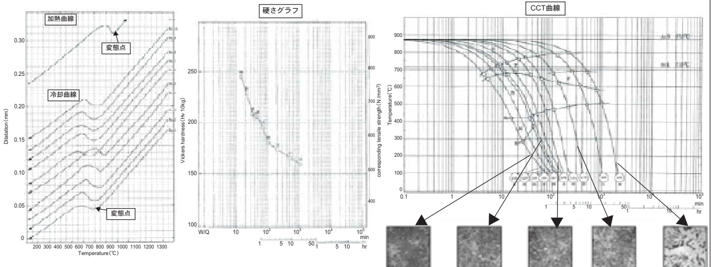
図1 連続冷却曲線図(CCT曲線図)
