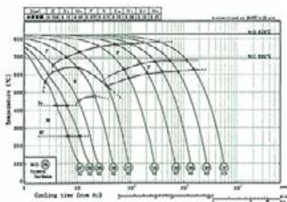
図2 C.C.T diagram
