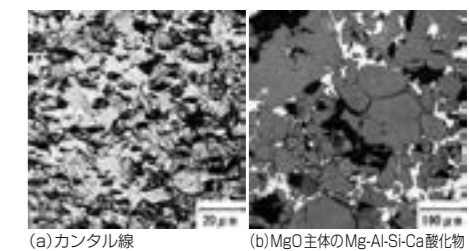
写真11 ヒーターに用いられる材料の光学顕微鏡写真
