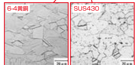
写真4 サーモスタット端子(6-4黄銅)、リード線(SUS430)と溶接部の光学顕微鏡写真
