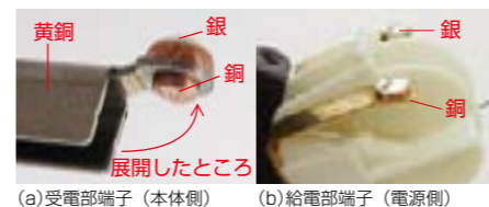
写真5 受電部と給電部の端子
