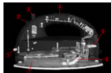
写真2 3D-X線CT画像による内部構造
