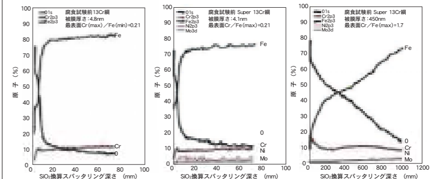
図4 ESCAによる腐食試験前後の表面被膜解析結果
