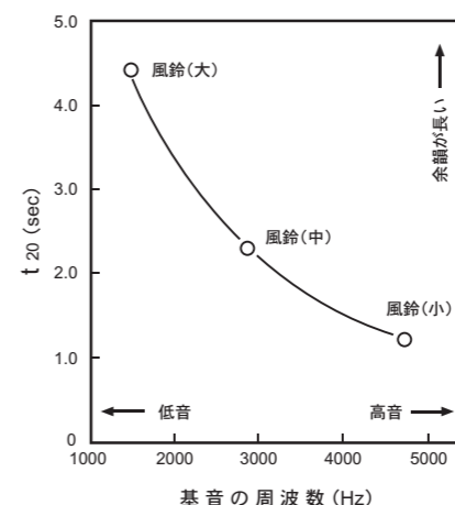
図5 基音の周波数と20dB減衰する時間
