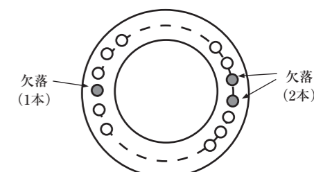
図8 ボルト欠落の影響
