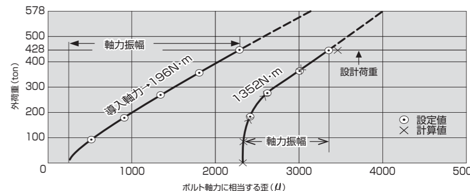
図7 ボルト導入軸力の影響
