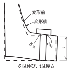
図5 てこ反力とボルトの曲げ
