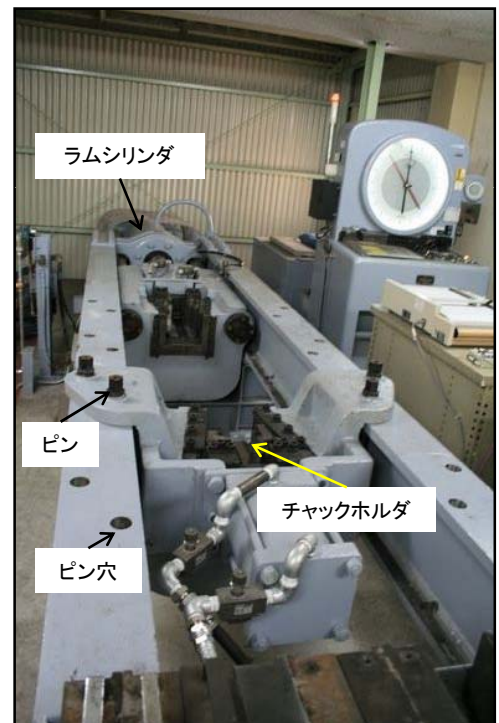
写真2 試験機全景
