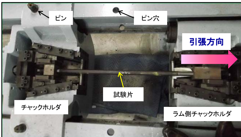
写真1 試験片掴み例
