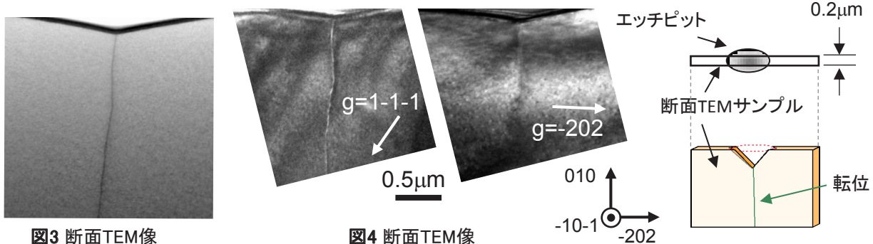
図3 断面TEM像
