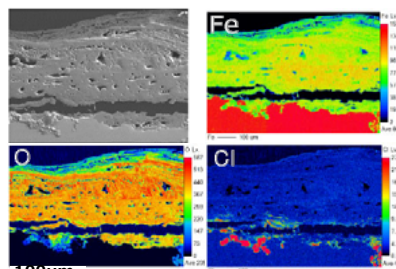
腐食断面分析(SM490C)
