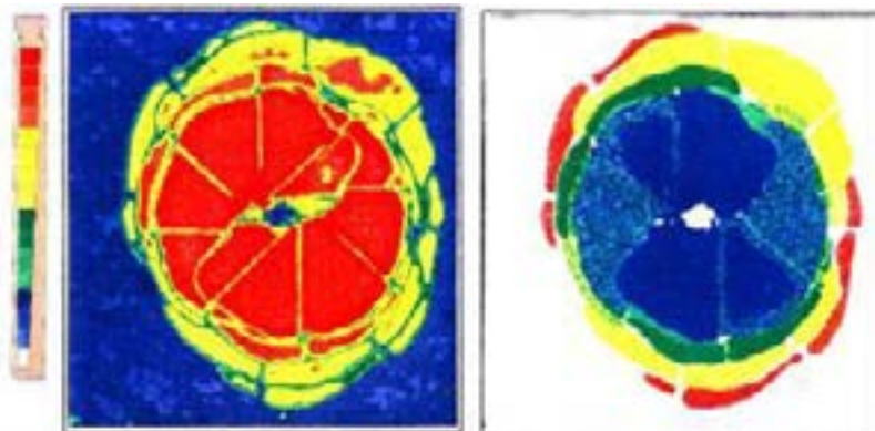
CFRP積層板の落錘試験後の剥離検査 (10mmtx50x50mm)
