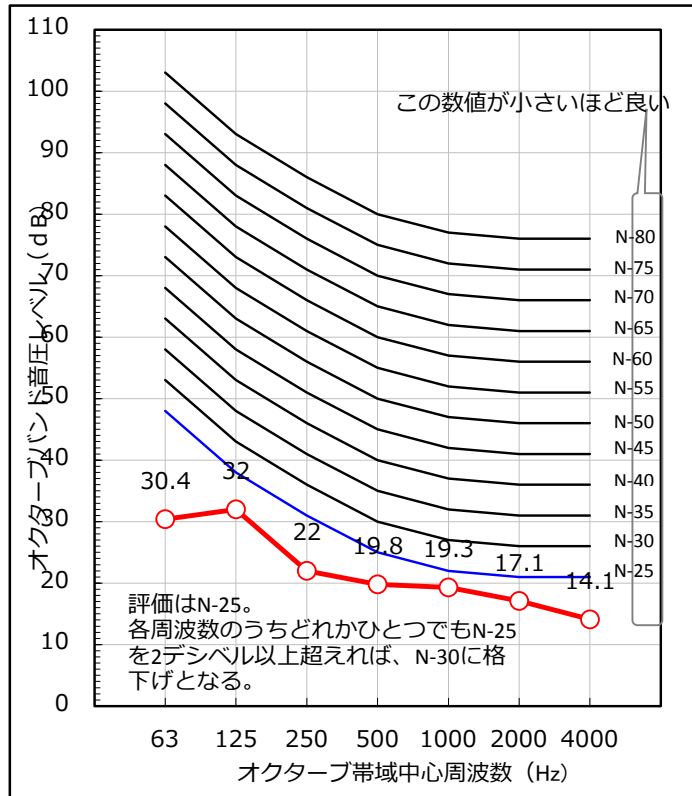
建物の内部騒音に関する騒音等級の基準周波数特性
