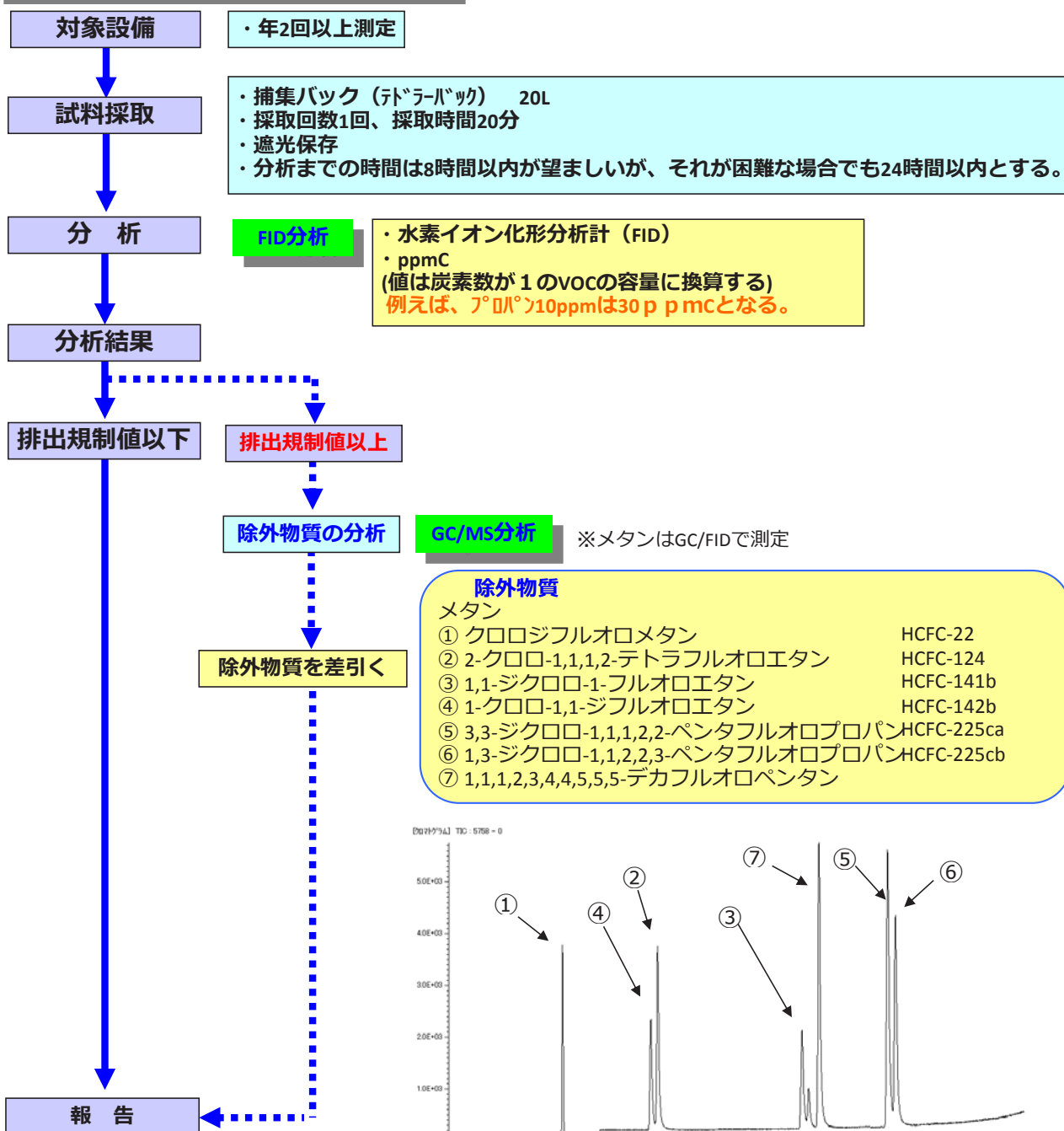
図 除外物質 (メタンを除く) のGC/MSによる分析例
