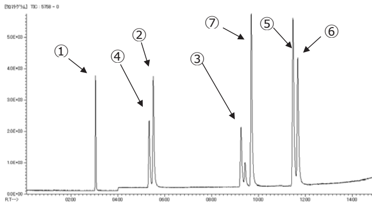
図 除外物質 (メタンを除く) のGC/MSによる分析例
