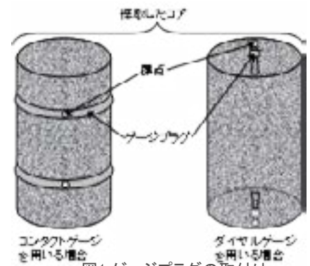
図1 ゲージプラグの取付け
