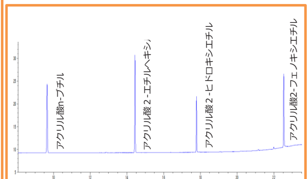
分析クロマトグラム
