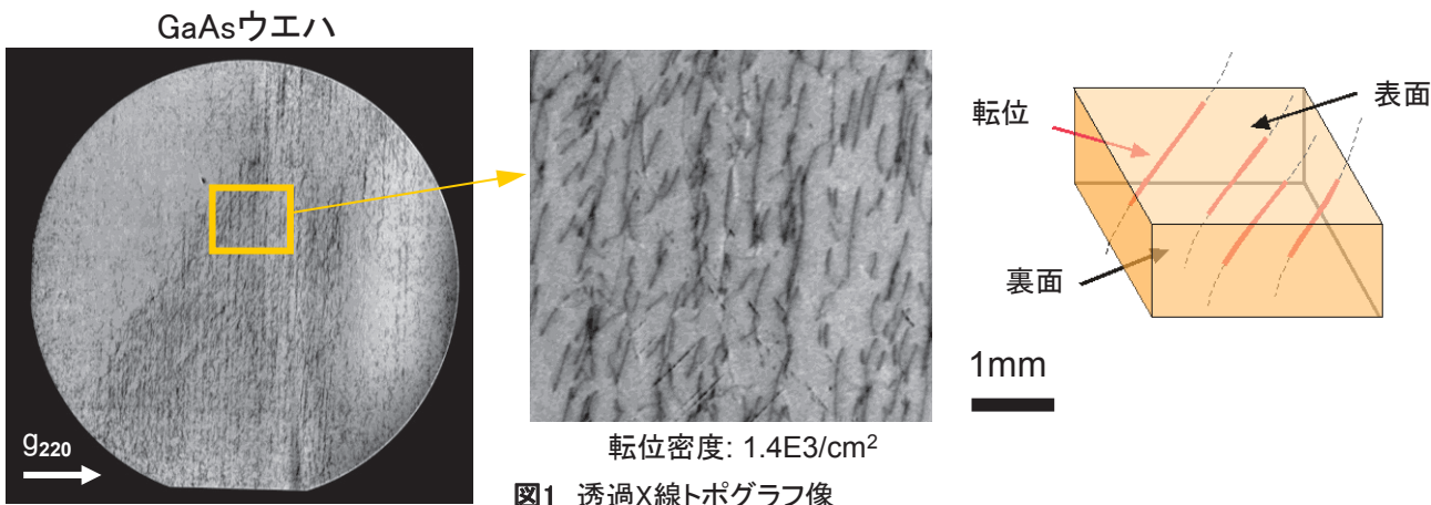
図1 透過X線トポグラフ像
