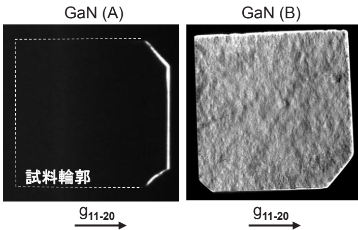
図2 透過X線トポグラフ像
